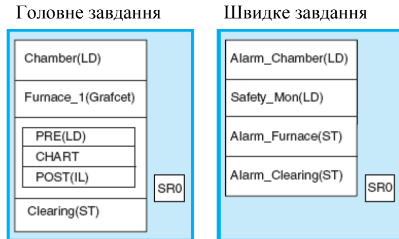
Рисунок 5.7 - Структури програма PL7
