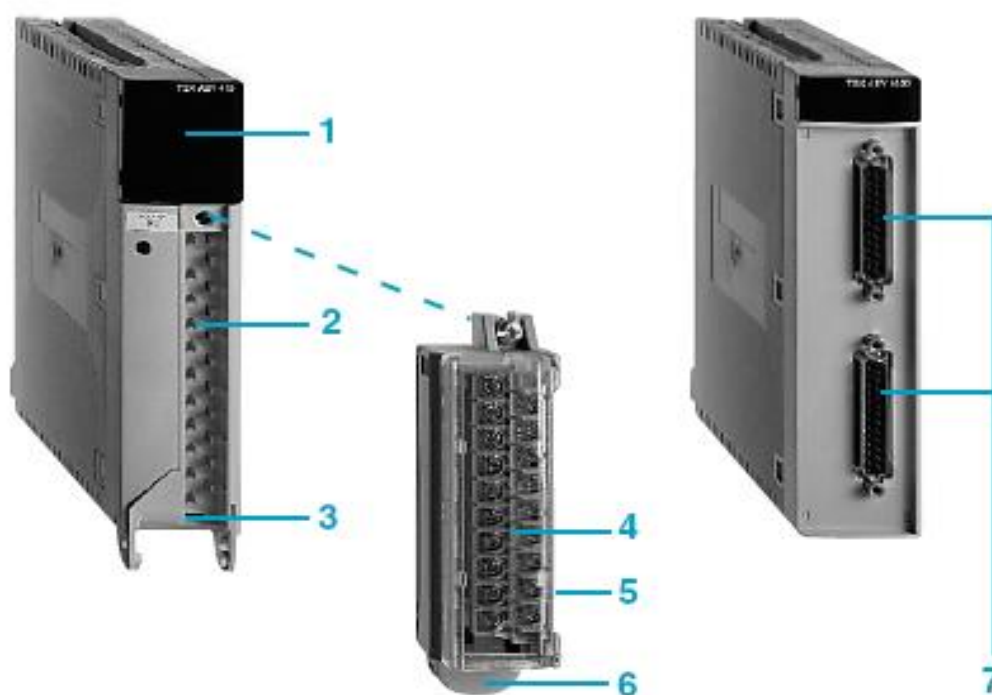
Рисунок 5.8 - Лицьова панель модулів TSX AEY/ASY
