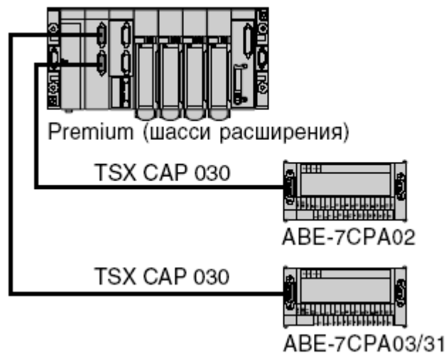
Рисунок 5.9 -Колодка Telefasі ABE-7CPA02 \ ABE7CPA03/31
