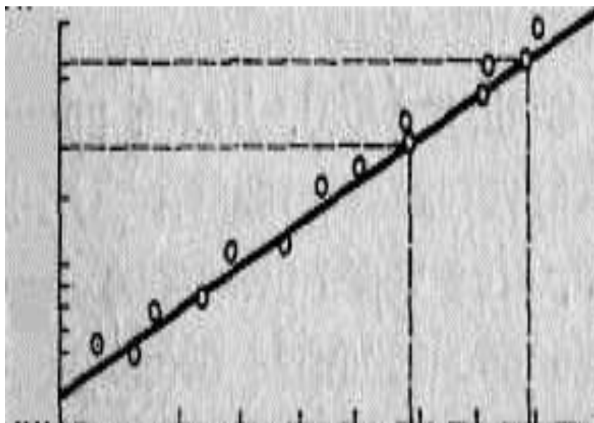
Рисунок 2.1 - Залежність електричного опору утфелю R від коефіцієнта пересичення a_{np}
