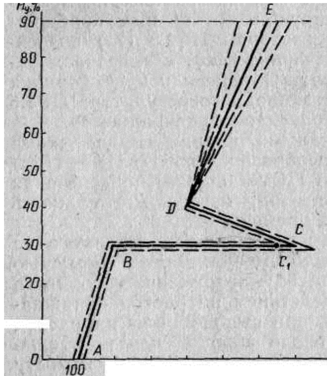
Рисунок 2.2 - Залежність між електричним опором утфелю R і його рівнем Ну у вакуум-апараті при уварюванні: АВ - ділянка наповнення апарату сиропом до рівня, що забезпечує повне покриття поверхні нагріву; ВСі - ділянка згущення сиропу до введення затравки; Сі - точка введення затравки; С 1 , С - ділянка утворення кристалів; CD - ділянка розкачки утфелю сиропом; DE - ділянку росту кристалів
